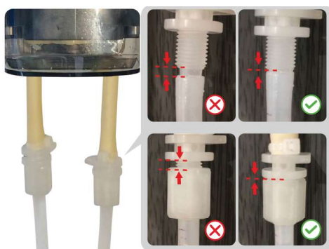
Figuur 4. Zure buis installatie
