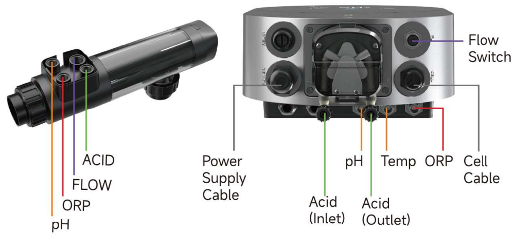
Figuur 1. Detail van sonde en interface
