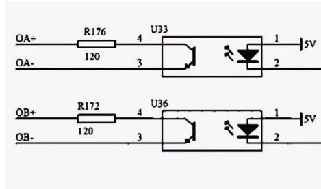
Figuur 20. OA+, OA-, OB+ en OB-
