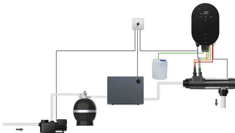
Figuur 3. Installatieschema
